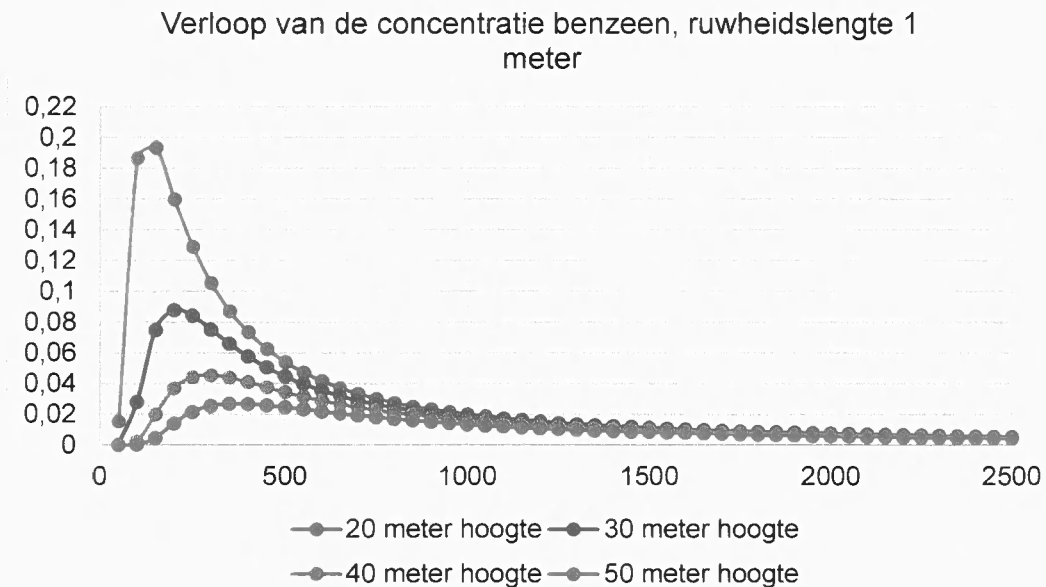
Figuur 3.2 Verloop van de jaargemiddelde benzeenconcentratie ( \mu\text{g}/\text{m}^3 ) bij een emissievracht van 500 g/uur en een ruwheidslengte van één meter
