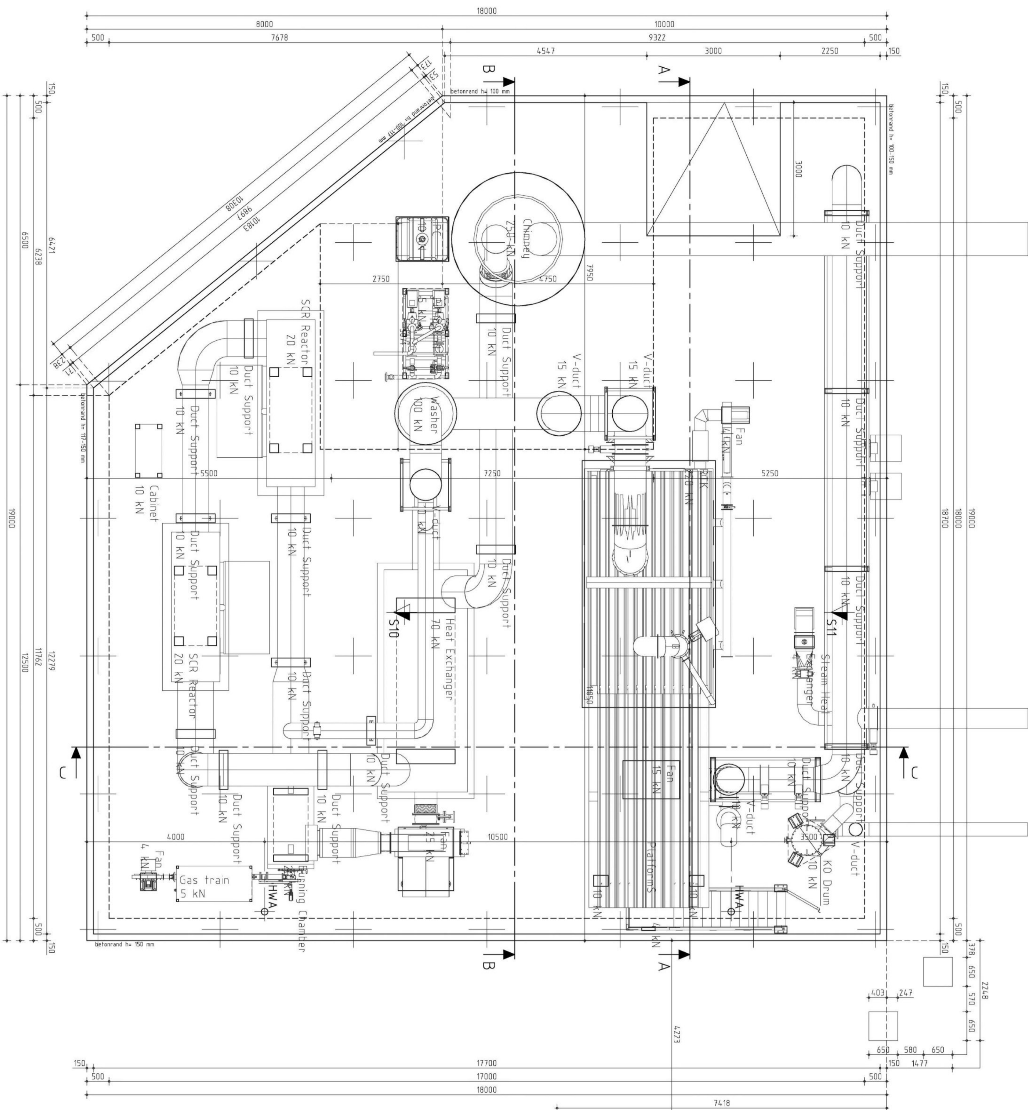
Bovenaanzicht betonplaat incl. belastingen
