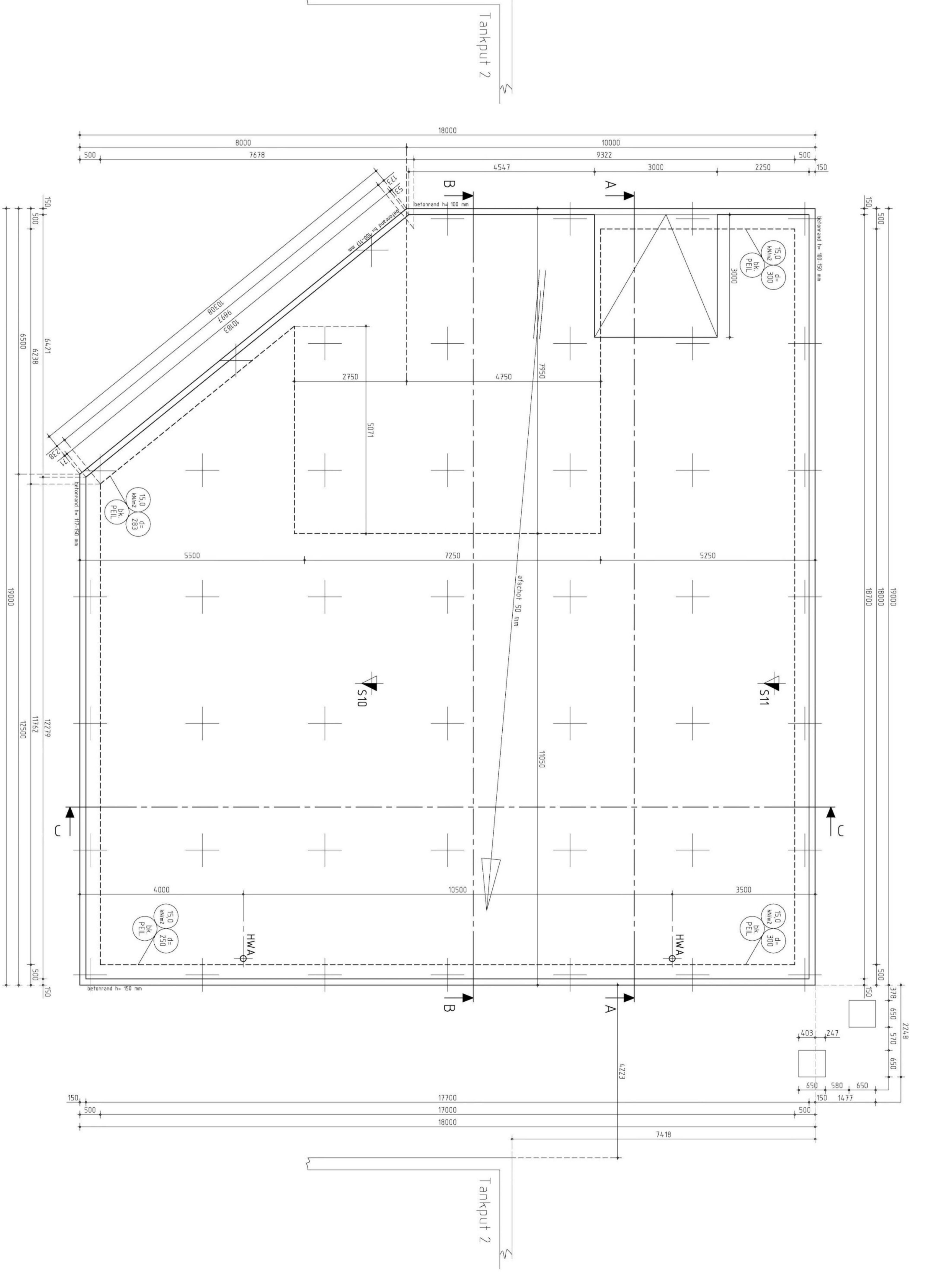
Vorm betonplaat
