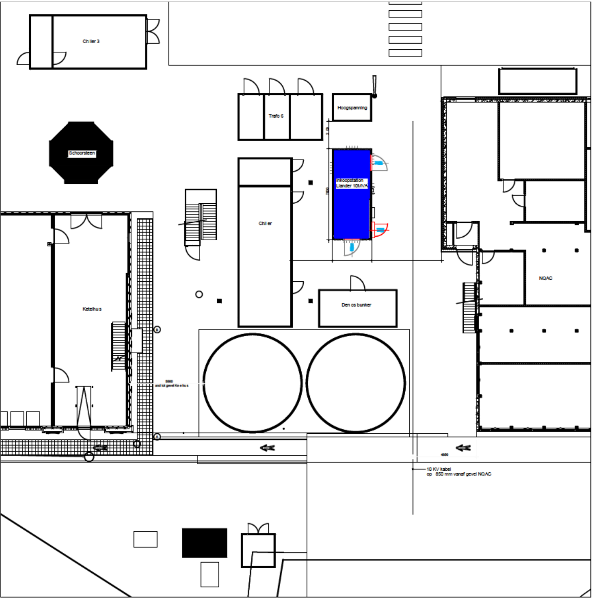
Begane grond gewijzigd 1 : 100
