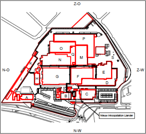
Situatie 1 : 2000
